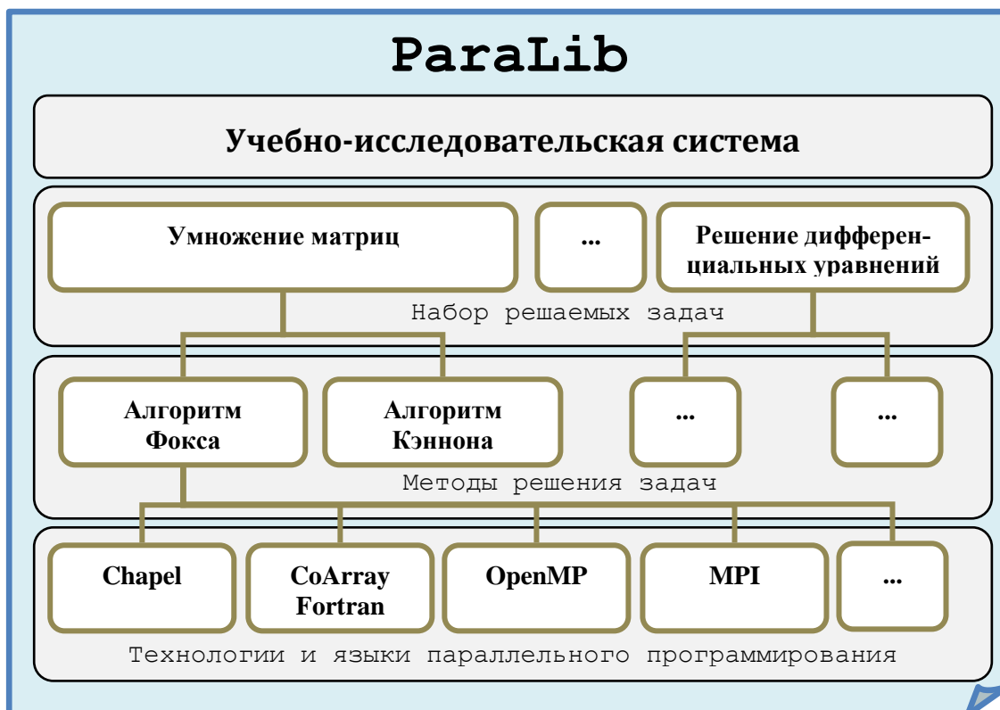
Рис. 5. Архитектура программного комплекса параллельных численных методов ParaLib
