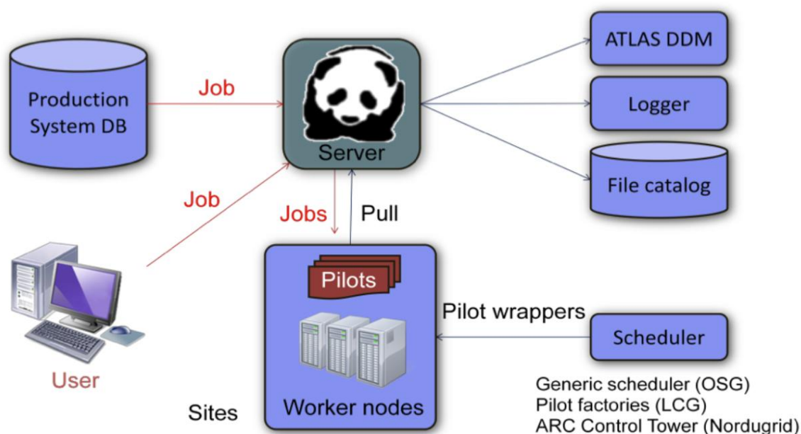
Рис. 1. Архитектура системы вычислений
