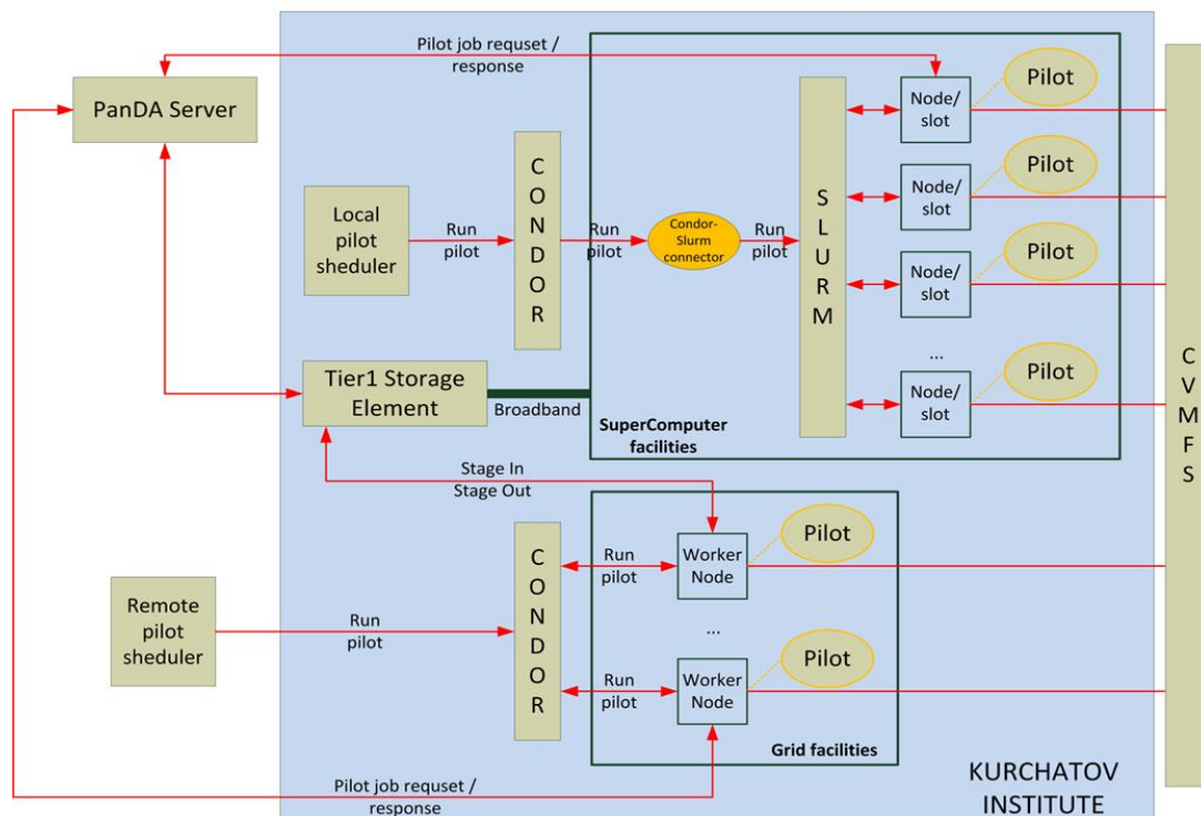
Рис. 2. Схема интеграции суперкомпьютера НИЦ “Курчатовский институт” и Tier-1
